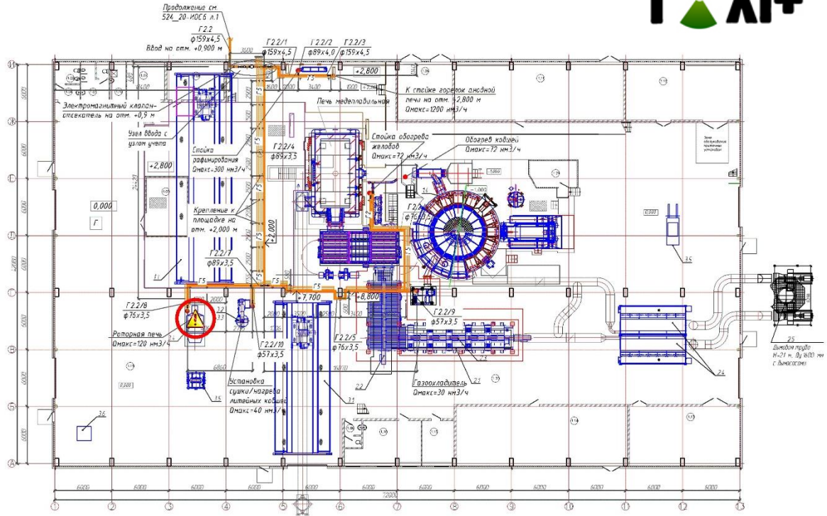
[REDACTED] Зона воздействия высокотемпературных продуктов сгорания Рисунок 8 – Ситуационный план для пожара вспышки для ситуации 4С2.1
