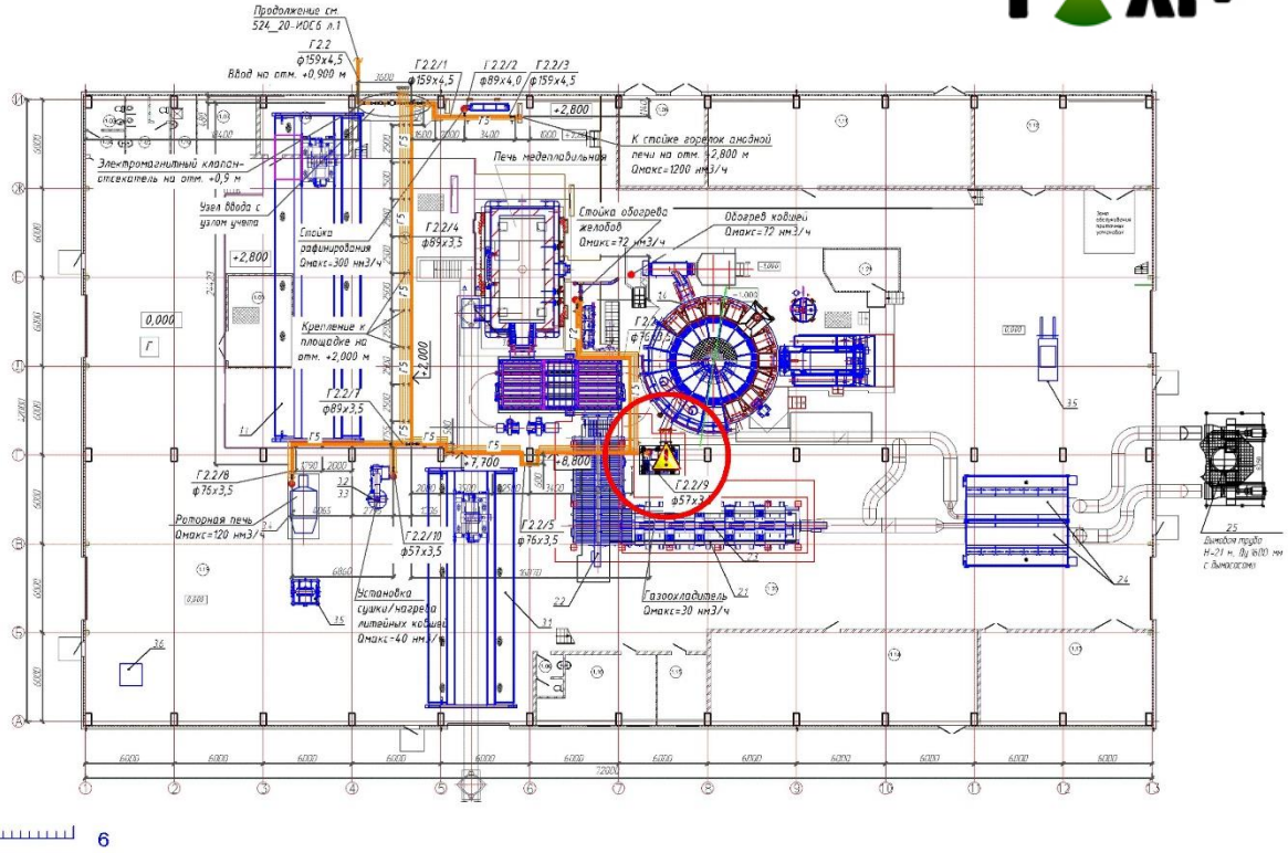
План внутренних газопроводов на отм. 0,000 м М1:200
