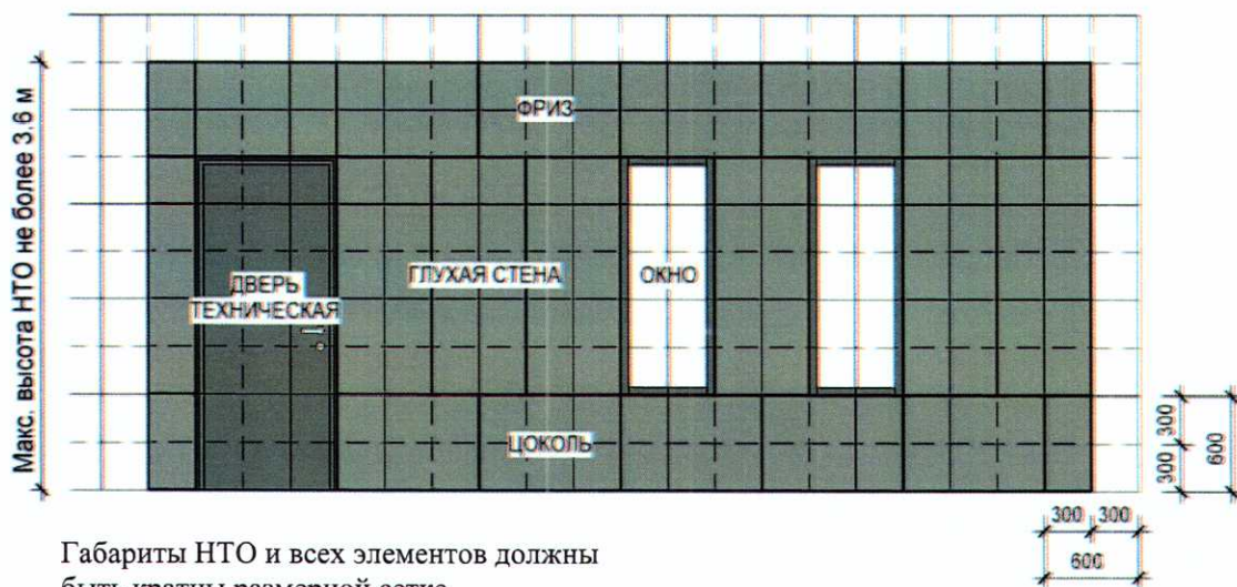
Задний и боковые фасады
