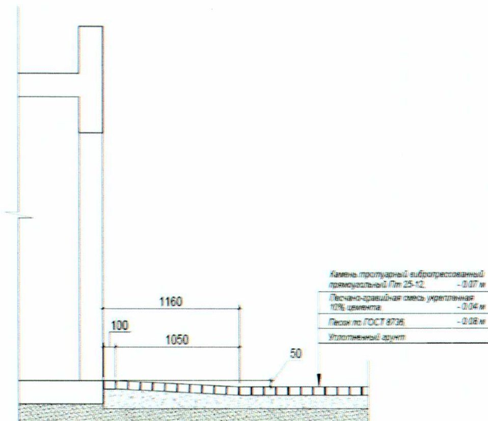
Схема повышения тротуара до уровня чистого пола НТО по периметру наружной
