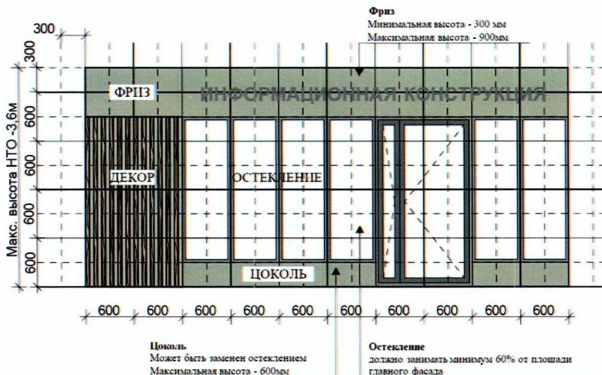
Задний и боковые фасады
