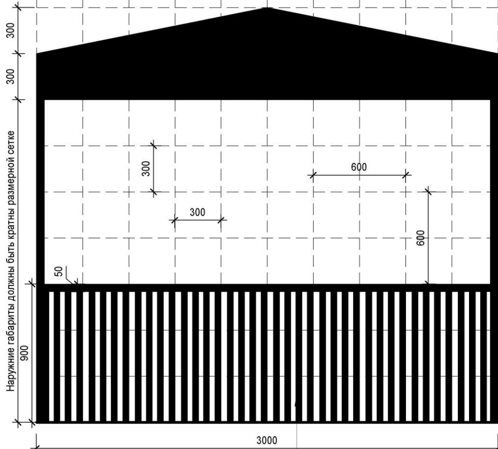
открытый с 1 стороны (возможен только при блокировке)
