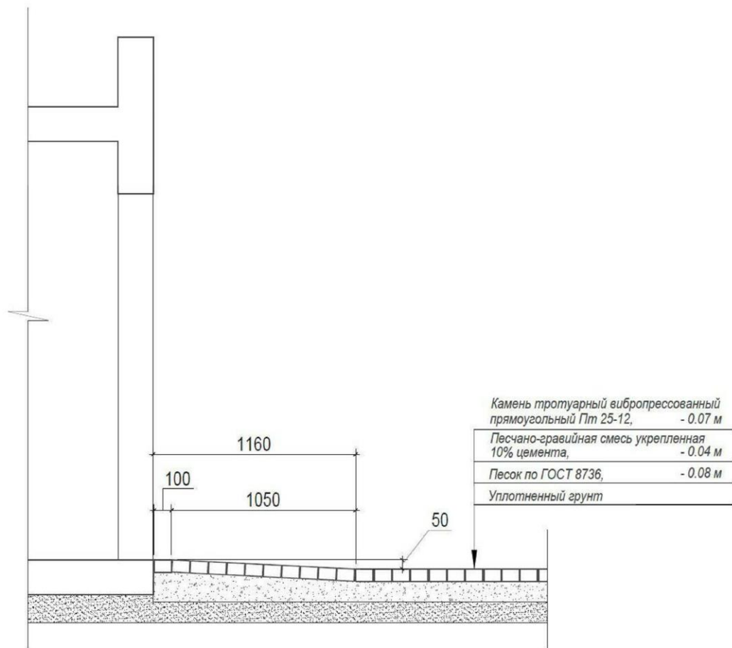
Схема повышения тротуара до уровня пола НТО по периметру наружной отделки
