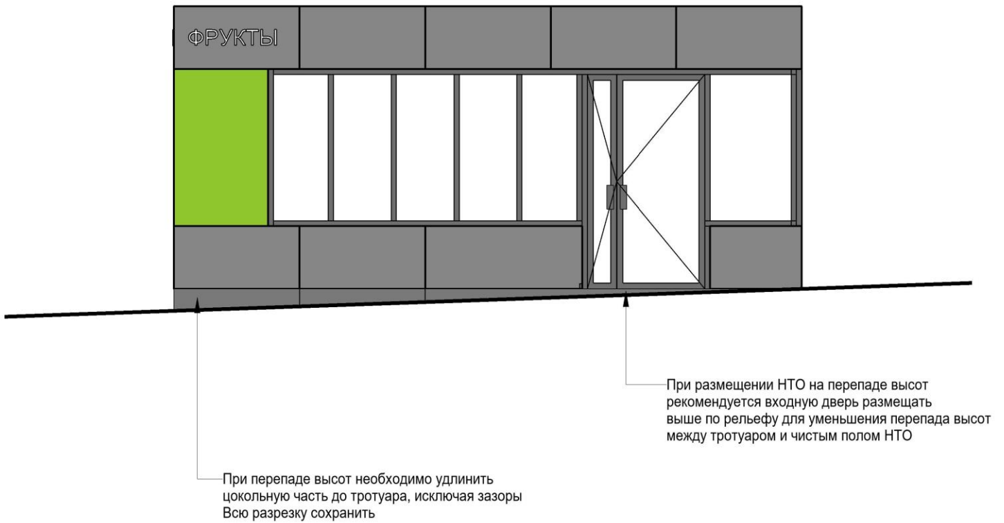
Схема повышения тротуара до уровня пола НТО по периметру наружной отделки
