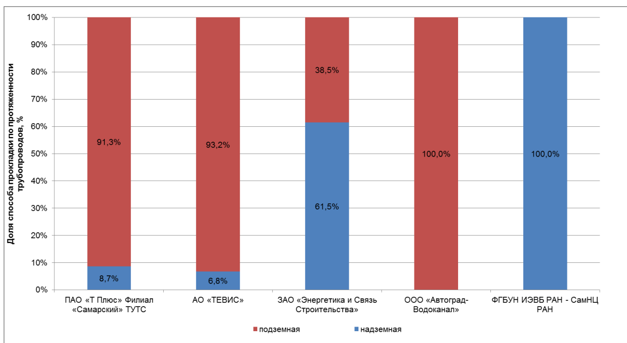
Рисунок 1.5 - Распределение долей способа прокладки по протяженности трубопроводов, %
