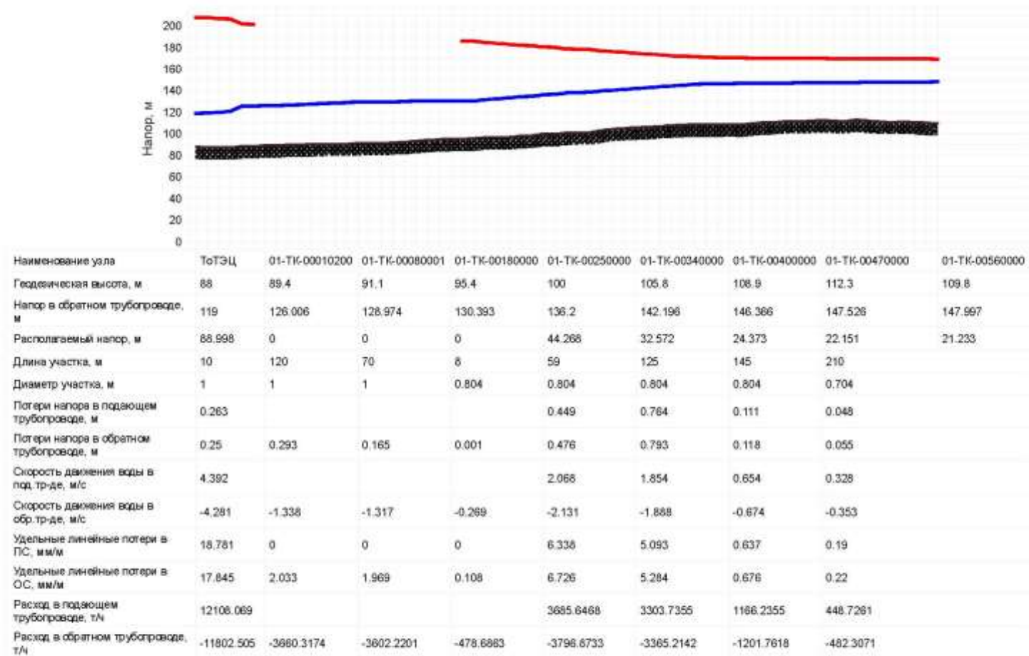
Пьезометрический график от «ТоТЭЦ» до «01-ТК-00560000»
