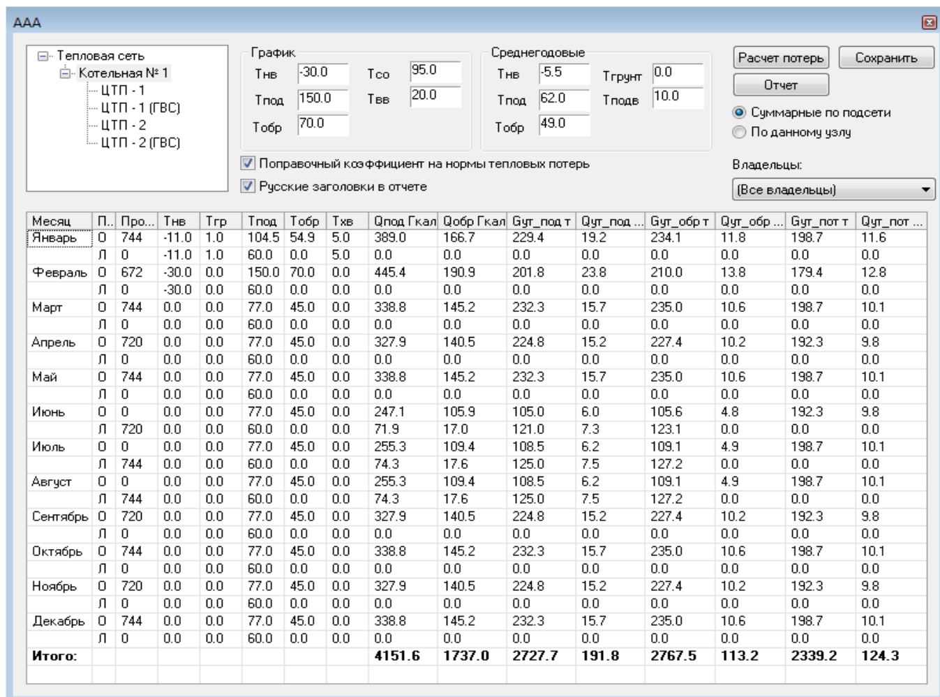
Рисунок 17 – Расчет тепловых потерь через изоляцию
