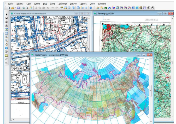
Рисунок 4 – Растровые данные
