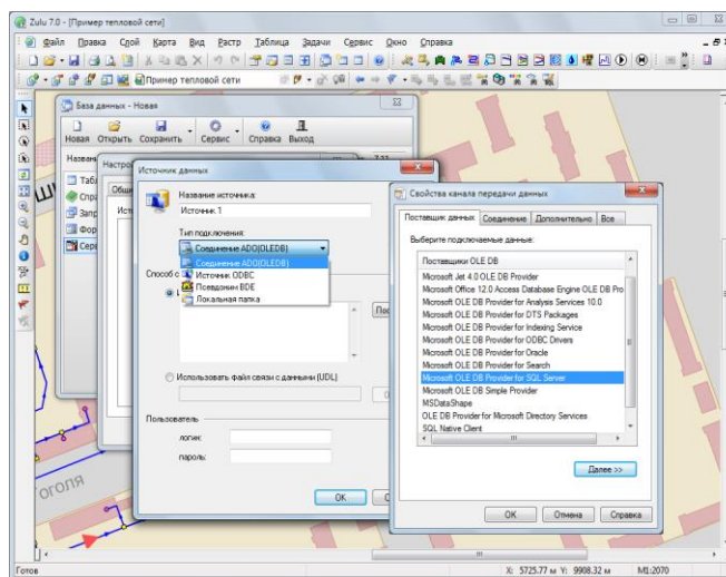
Рисунок 6 – Семантическая информация
