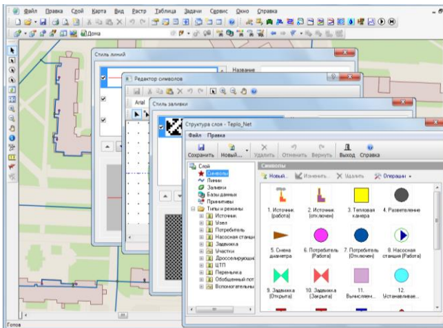
Рисунок 3 – Векторные данные
